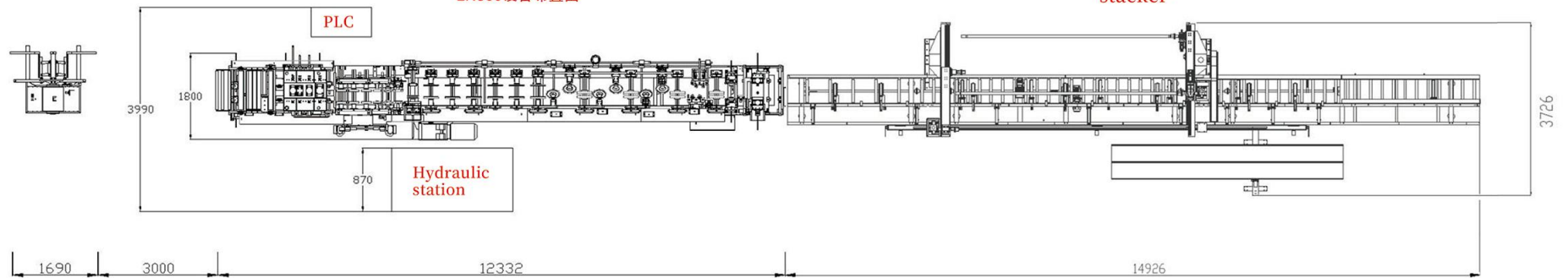
LN300设备布置图
